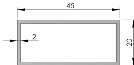
PERFIL 45x20
