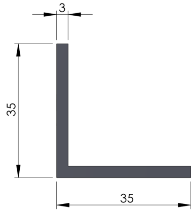
PERFIL L 35x35X3
