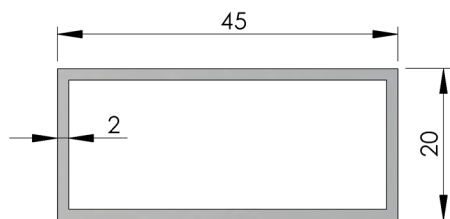
PERFIL 45x20
